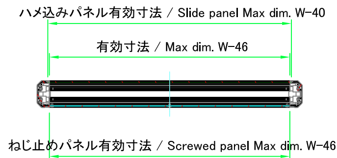
A-A ( 1 : 7 )
