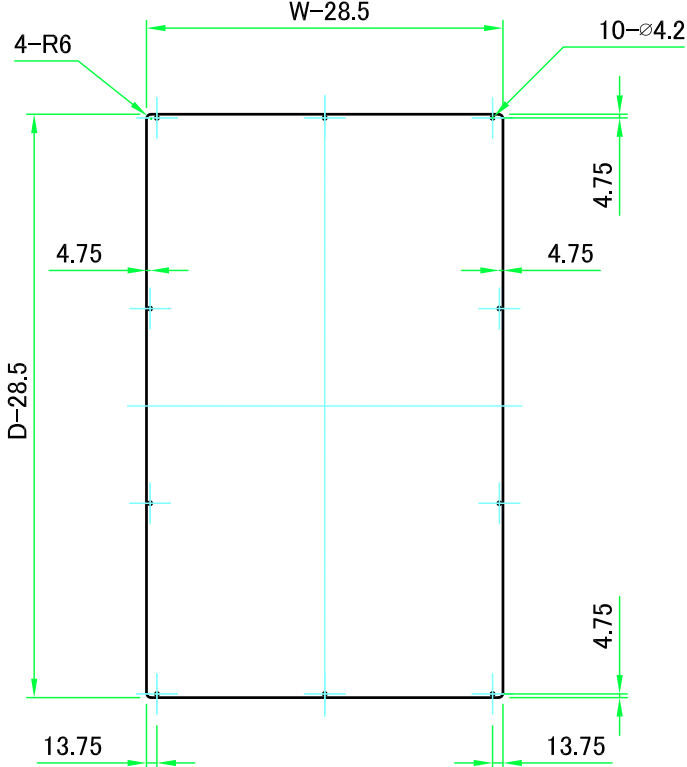
パネル裏面 / Panel Backside
